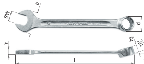
DIN 3113 Shape A
